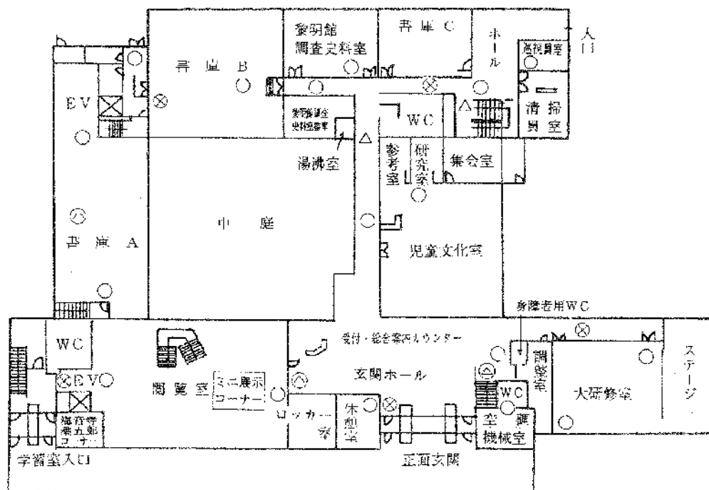
本館 1 階 平面図
